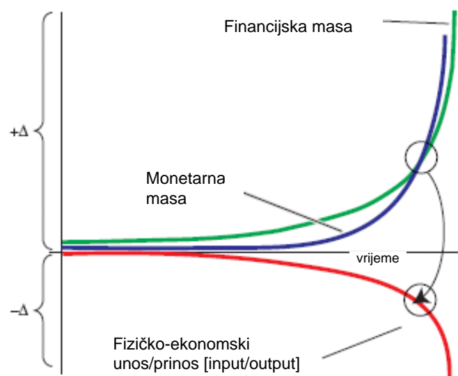
Prikaz 2 Pad dosiže kritičnu točku nestabilnosti
