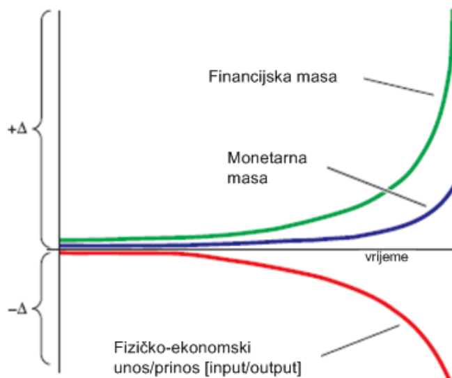
Prikaz 1 LaRouche-eva Trostruka krivulja
